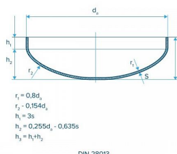
DIN 28013
